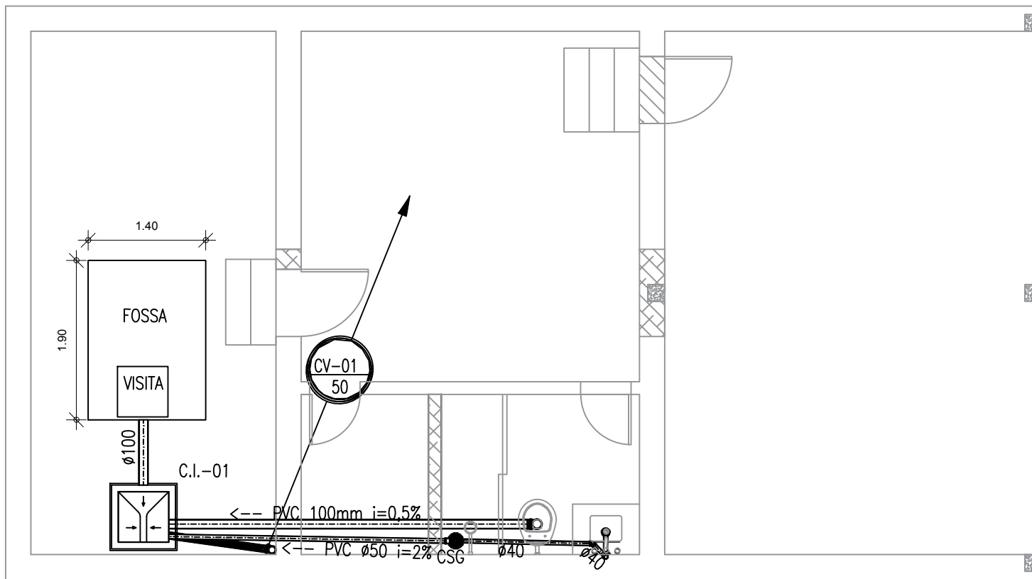
01 - PLANTA BAIXA - SANITÁRIO escala: 1/50
