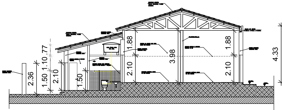
2 CORTE C ESCALA _____ 1:100
