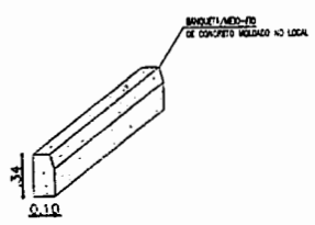
MEIO-FIO (3D) ESCALA 1/30
