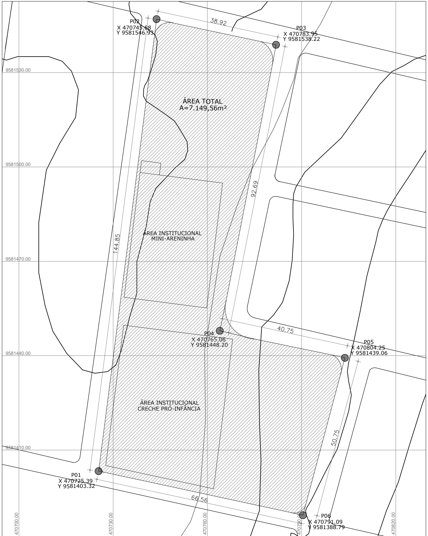
01/PLANTA DE SITUAÇÃO GEORREFERENCIADA esc. 1:750
