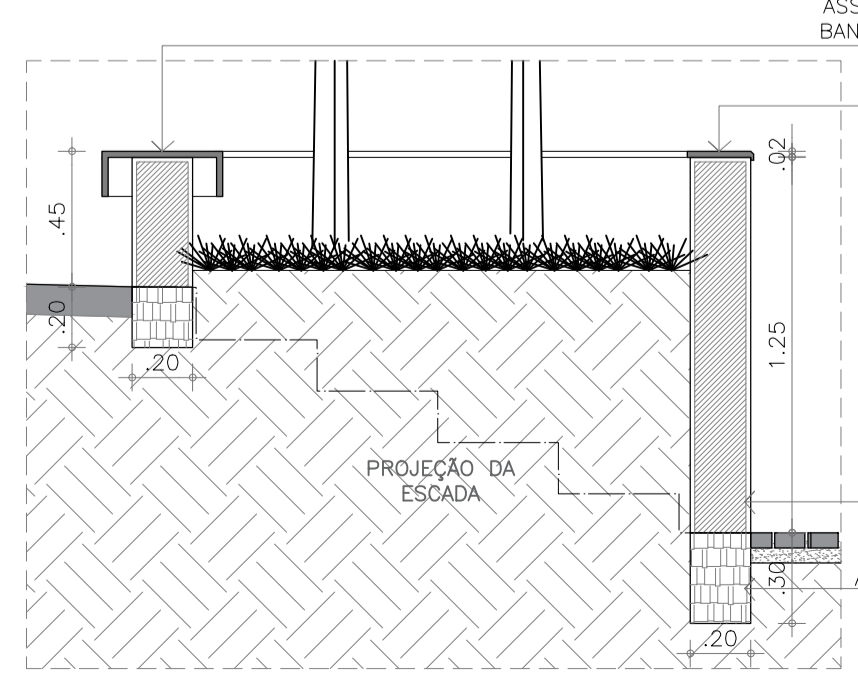
D1/DETALHE 01 - CANTEIRO esc.: 1:25
