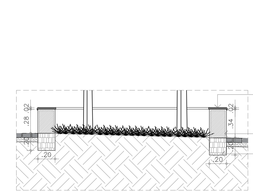
D2/DETALHE 02 - CANTEIRO esc.: 1:25
