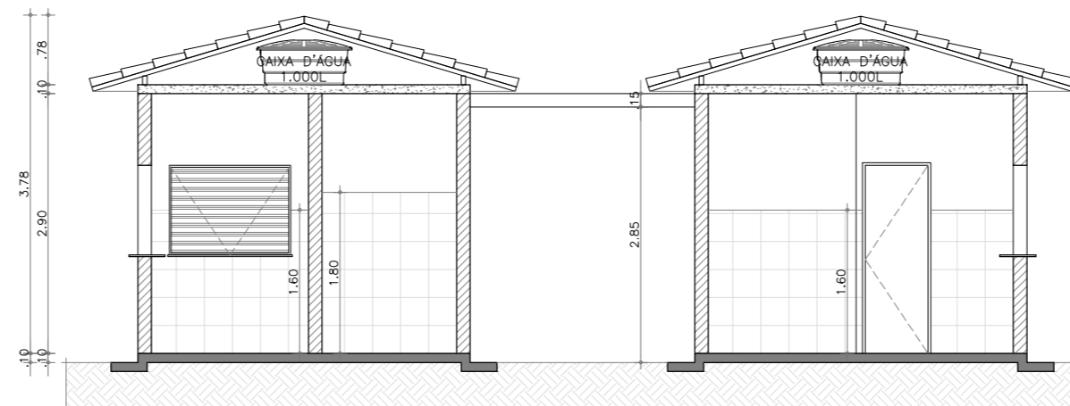
CC/CORTE CC esc. 1/75
