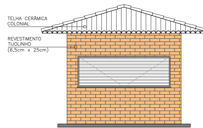
V1/VISTA 01 esc. 1/75
