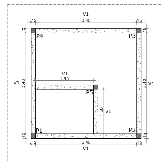
06/FORMAS E VIGAS SUPERIORES esc. 1/75
