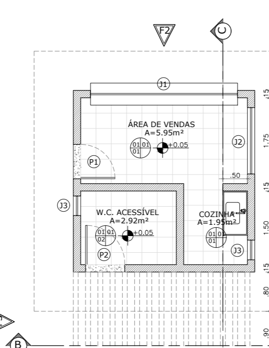
02/PLANTA - QUIOSQUE SIMPLES esc. 1/75
