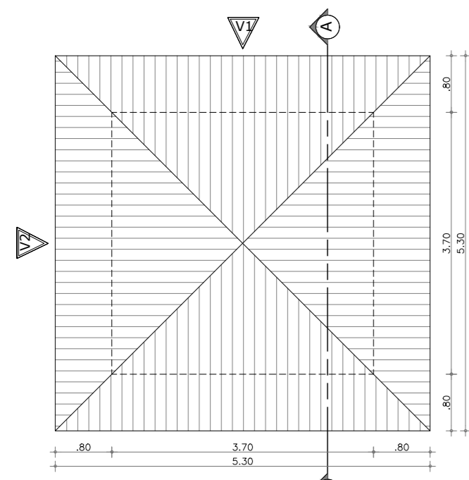
01/COBERTA - QUIOSQUE SIMPLES esc. 1/75
