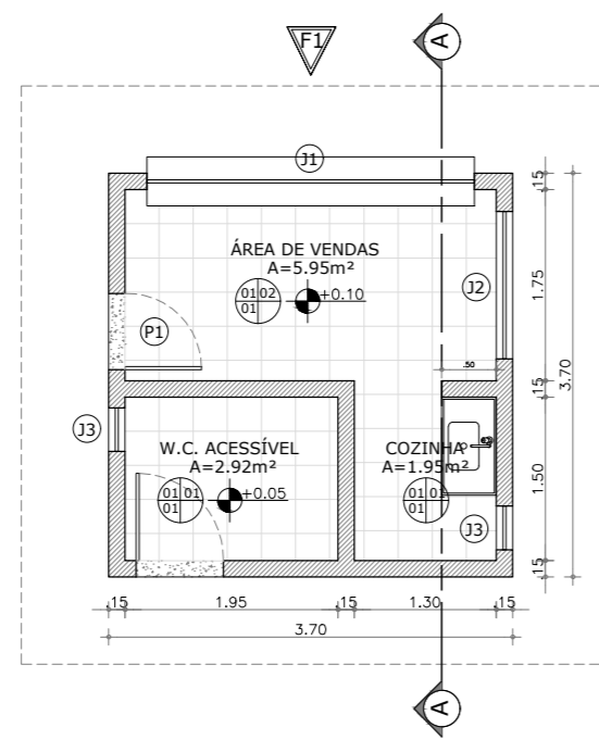
02/PLANTA - QUIOSQUE SIMPLES esc. 1/75
