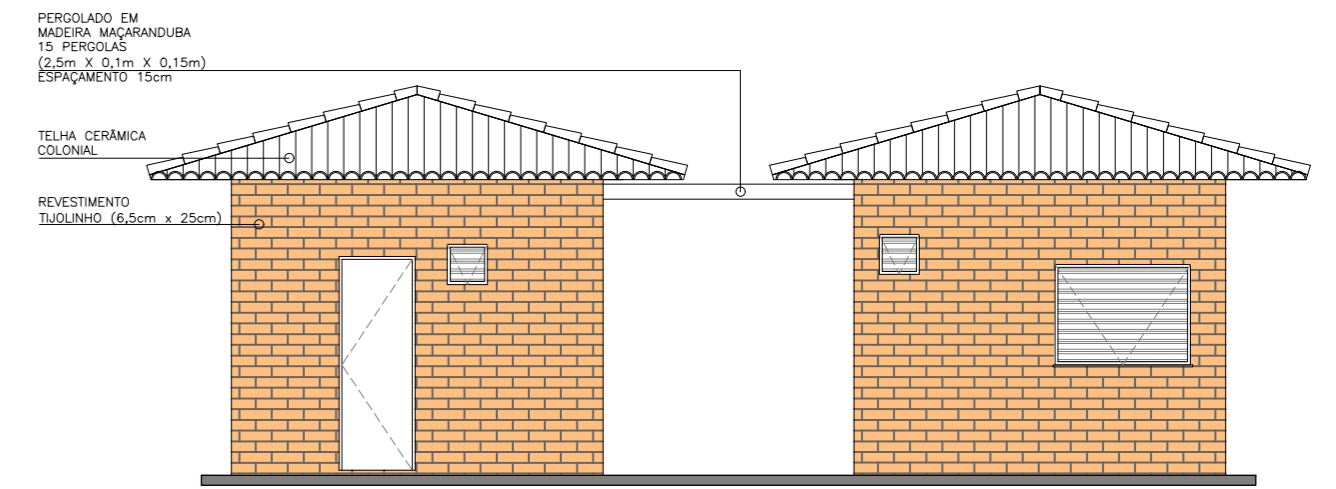
V4/VISTA 04 esc. 1/75
