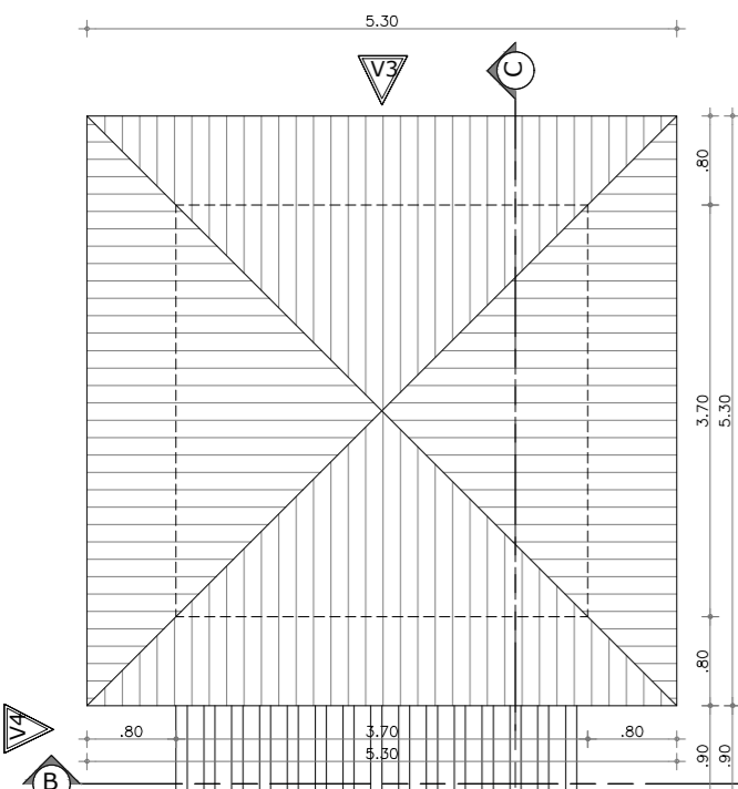
01/COBERTA - QUIOSQUE SIMPLES esc. 1/75
