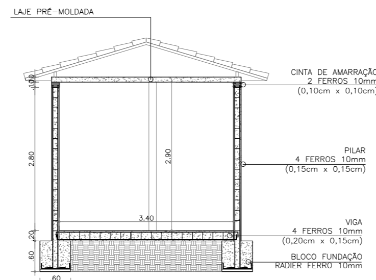
06/CORTE ESTRUTURAL esc. 1/75
