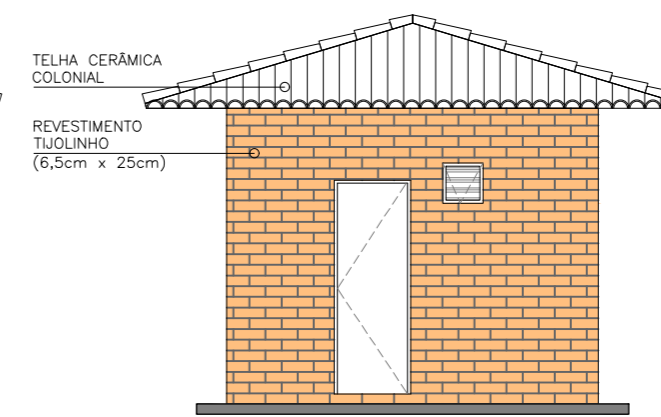
V2/VISTA 02 esc. 1/75
