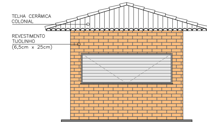
V3/VISTA 03 esc. 1/75
