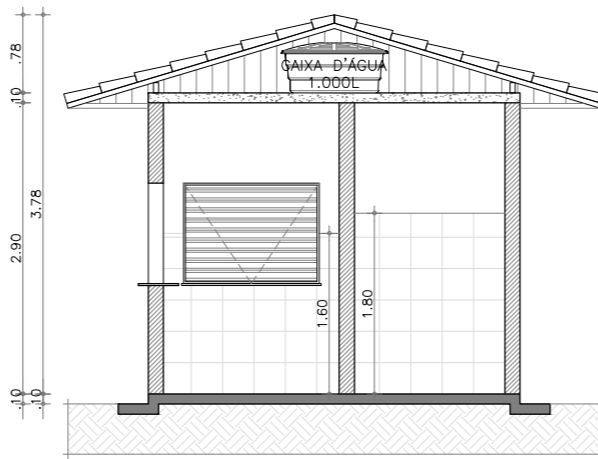
AA/CORTE AA esc. 1/75
