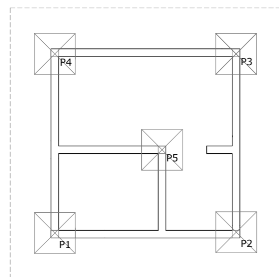
05/FUNDAÇÃO E VIGAS INFERIORES esc. 1/75
