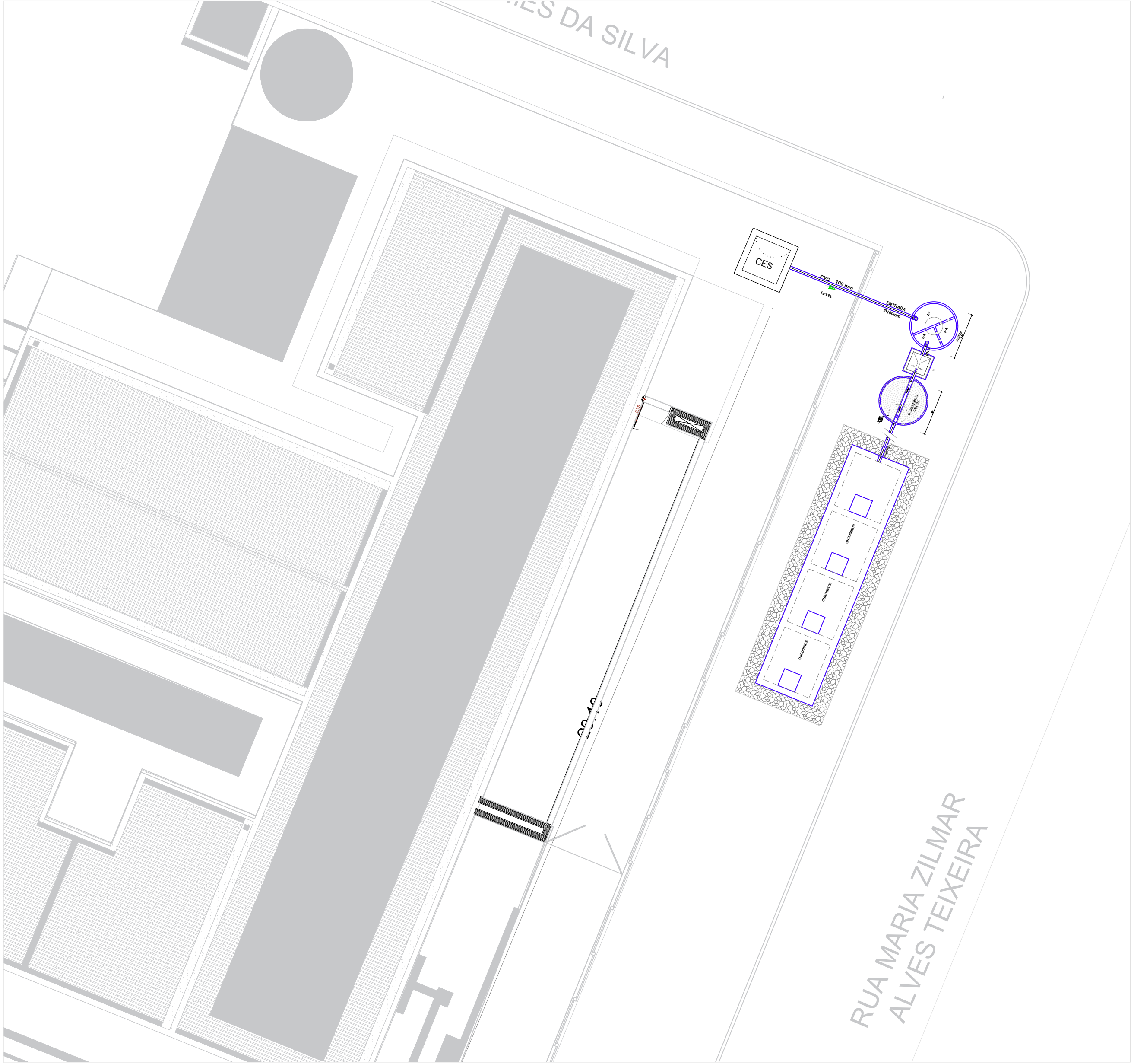
PLANTA LOCALIZAÇÃO - SISTEMA FOSSA / FILTRO/ SUMIDOURO ESC. 1/75
