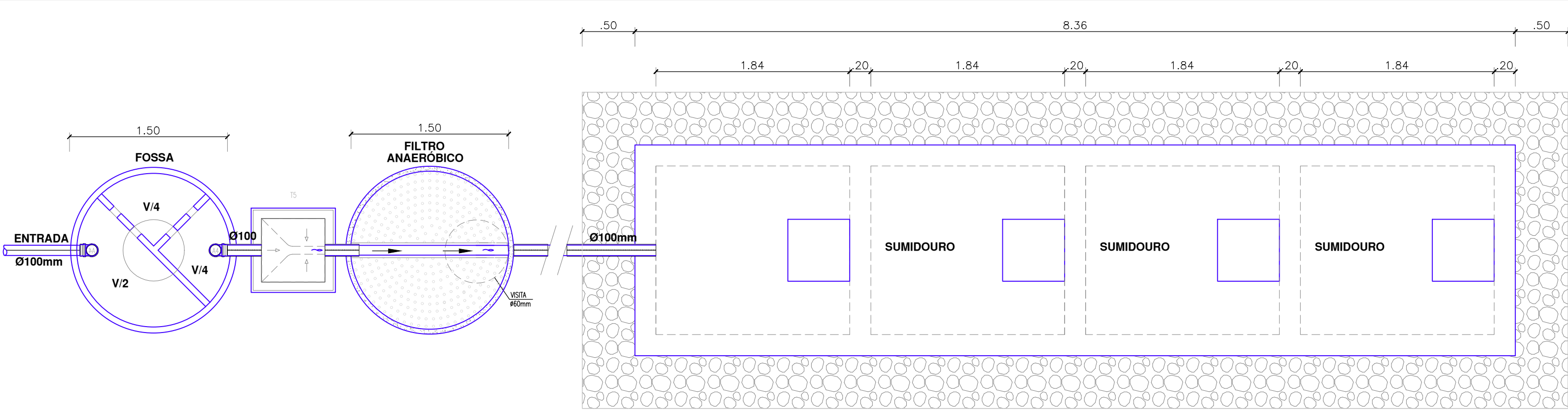
PLANTA CORTE - SISTEMA FOSSA / FILTRO/ SUMIDOURO ESC. 1/25
