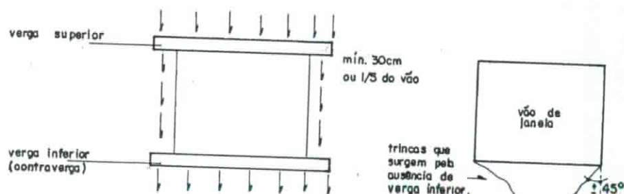
Figura 3 - Vergas sobre e sob os vãos.
